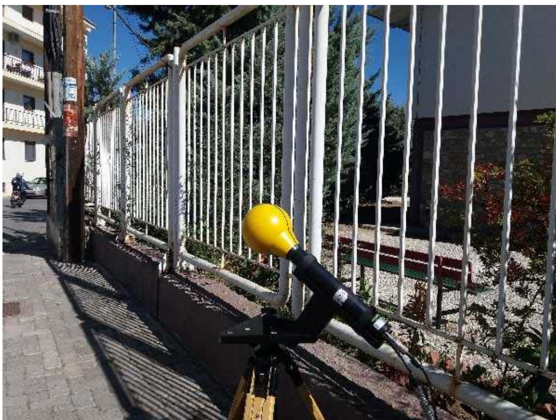
Εικόνα 7: Φωτογραφία που έχει ληφθεί κατά τη μέτρηση στο Σημείο 5.
