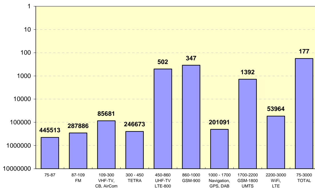
Εικόνα 10: Παράγοντας που δείχνει πόσες φορές χαμηλότερος από το όριο είναι ο Λόγος Έκθεσης σε κάθε υποπεριοχή του φάσματος 75 MHz – 3 GHz (Σημείο 2). Τιμή του παράγοντα μικρότερη από 1 δείχνει ότι η τιμή του Λόγου Έκθεσης δεν υπερβαίνει το όριο.
