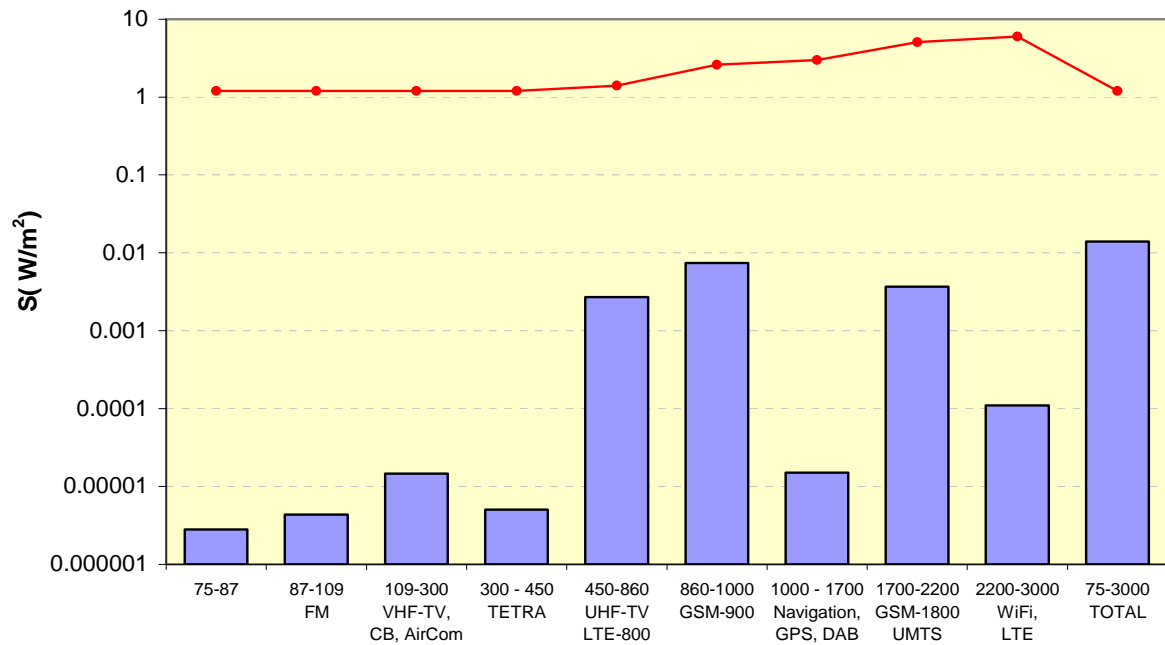
Εικόνα 11: Παράγοντας που δείχνει πόσες φορές κάτω από το όριο βρίσκεται η Πυκνότητα Ροής Ισχύος σε κάθε υποπεριοχή του φάσματος 75 MHz – 3 GHz (Σημείο 2). Ως όριο λαμβάνεται το 60% επί της αντίστοιχης τιμής του διεθνούς ορίου, σύμφωνα με την ισχύουσα Ελληνική νομοθεσία.
