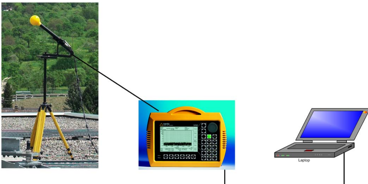
Εικόνα 2: Εξοπλισμός μετρήσεων.
